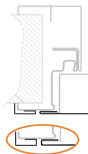
Eck-/Gegenzarge (Dünn-/Dickfalztür)
