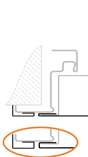
Eckzarge (Dünn-/Dickfalztür)
