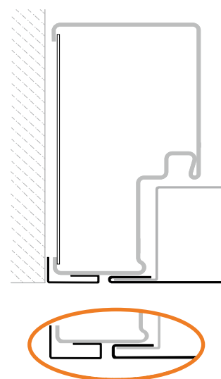
Blockzarge Typ 4.1 (Dünn-/Dickfalztür)
