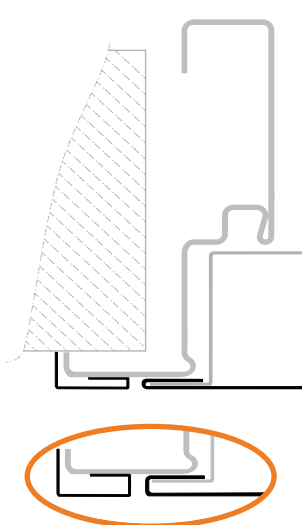
Umfassungszarge (Dünn-/Dickfalztür)
